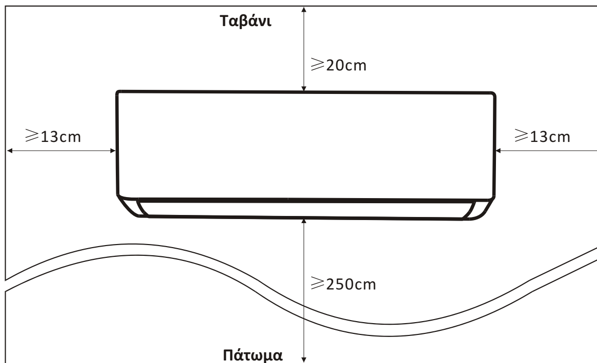
Ελάχιστες απαιτούμενες αποστάσεις εγκατάστασης εσωτ. μονάδας
